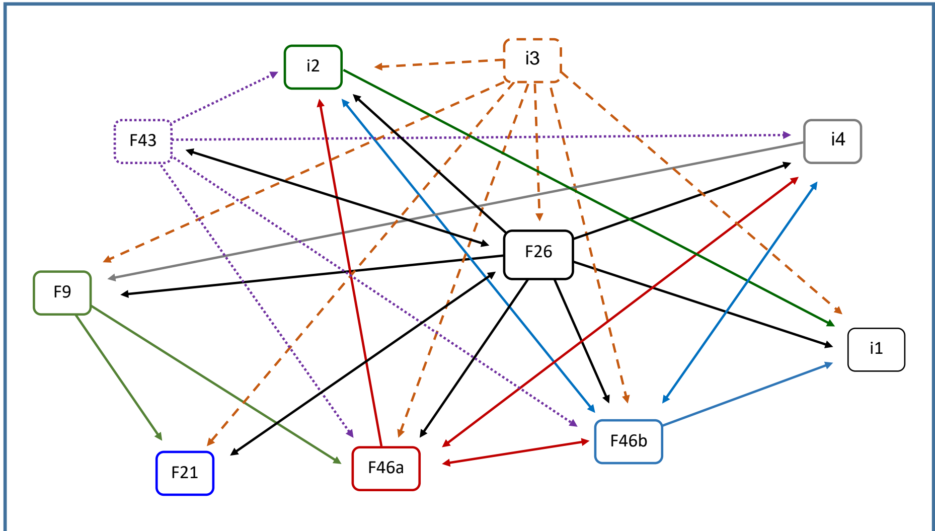
Abb. 4: Empirisches Kausalmodell von 10 unabhängigen Variablen aus Abbildung 3 (S. 63) und Tabelle 1 (S. 65) – Legende umseitig
