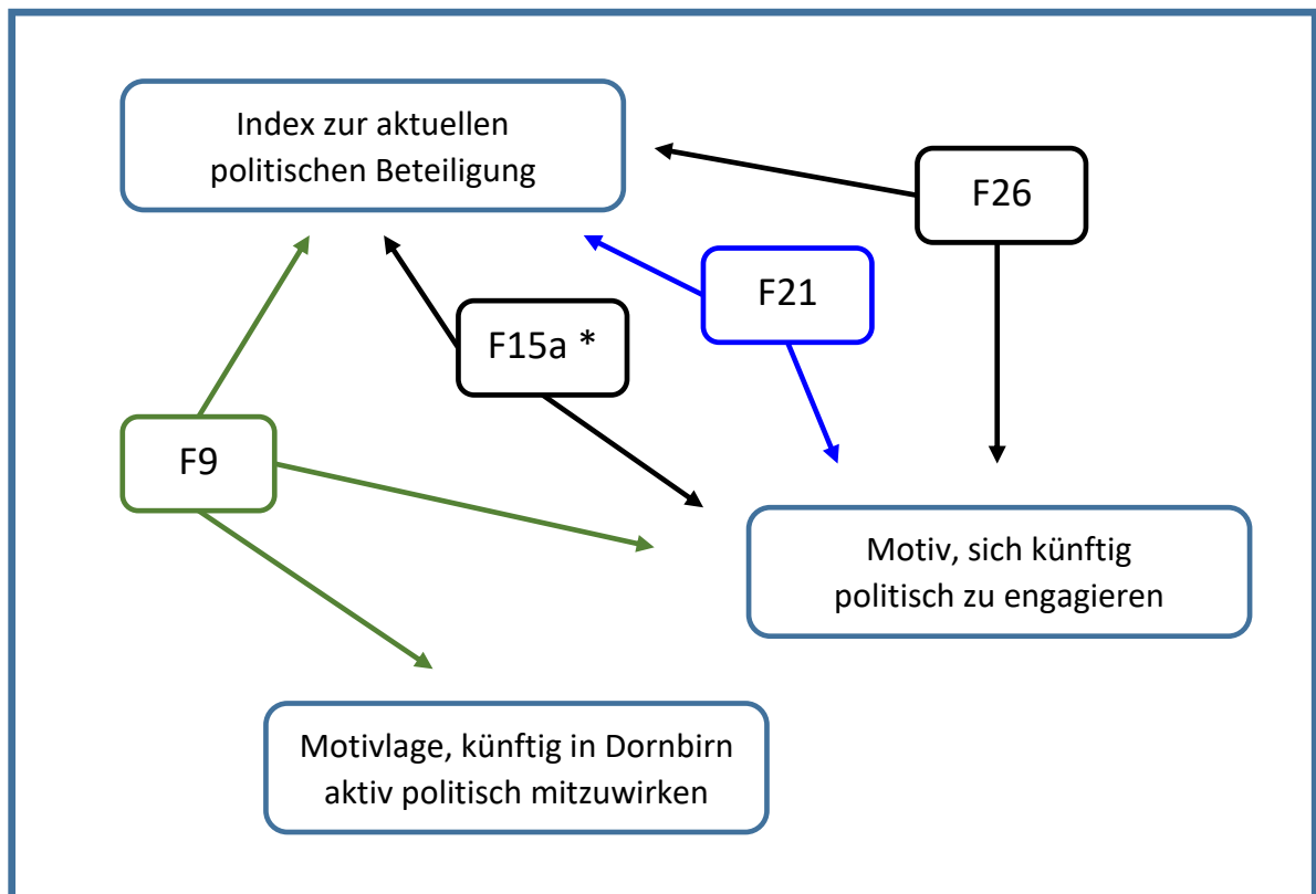
Abb. 4: Empirisches Kausalmodell von 13 unabhängigen Variablen aus Tabelle 2 (S. 66) auf aktuelle und potentielle politische Beteiligung
